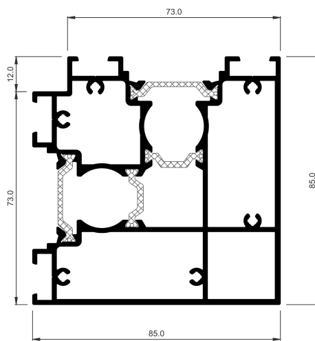
COR-3760 90° Corner
